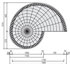
Εικόνα: Είσοδος δεξιά Πάχος στοιχείου δαπέδου: 50 mm
